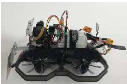
小型ドローン搭載試作機
